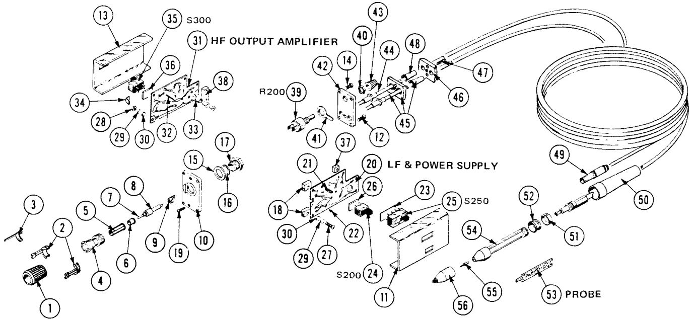
Fig. 6-1 P6201
